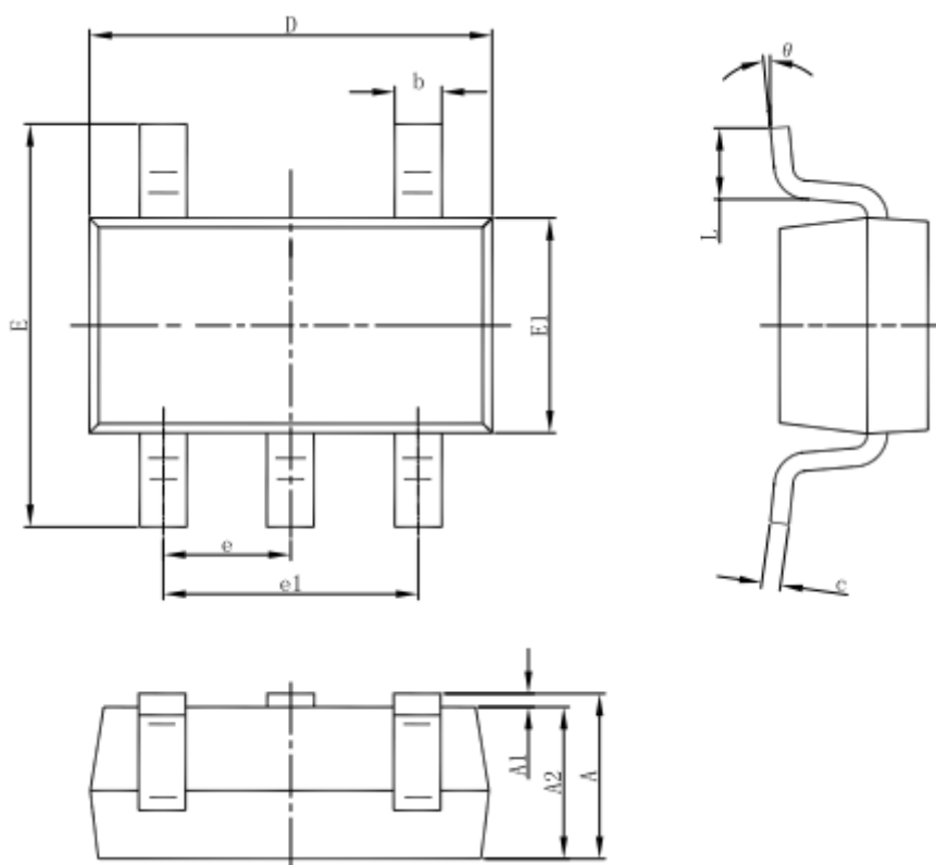
SOT23-5
